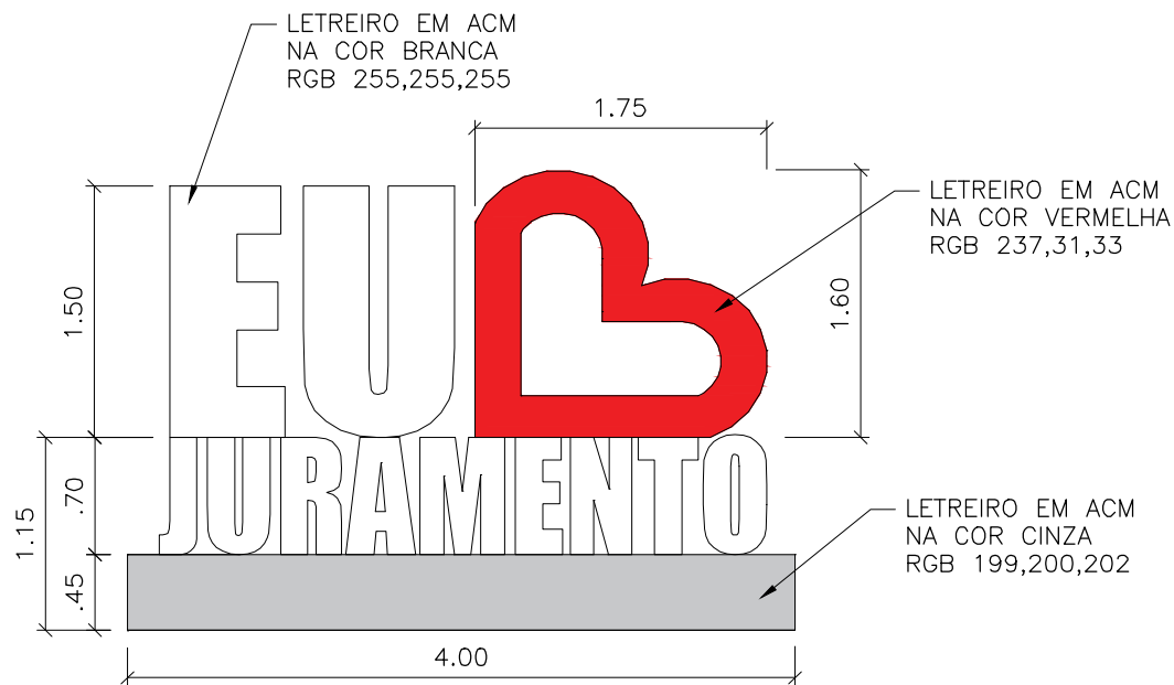
8 VISTA FRONTAL - LETREIRO ESCALA 1:50
