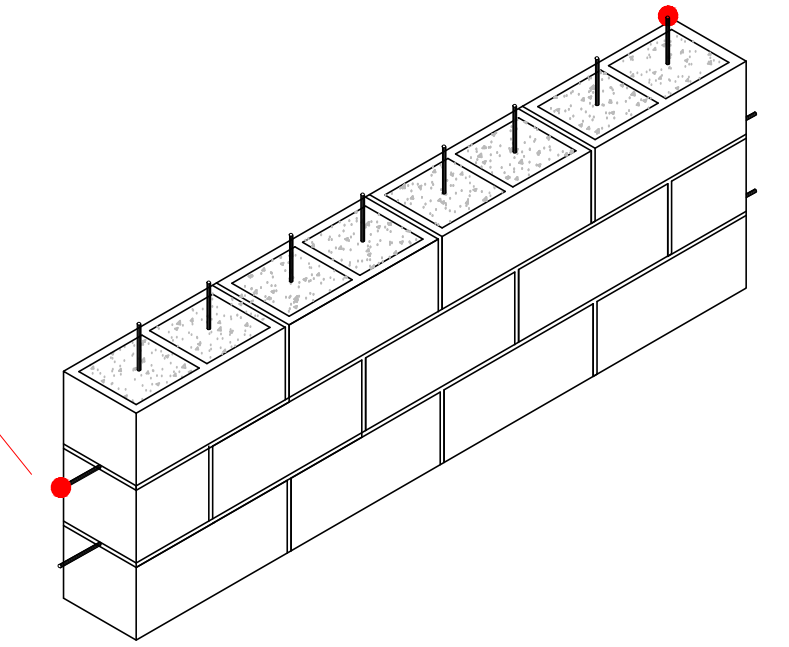
2 DETALHE DO BLOCO ARMADO ESCALA 1:50
