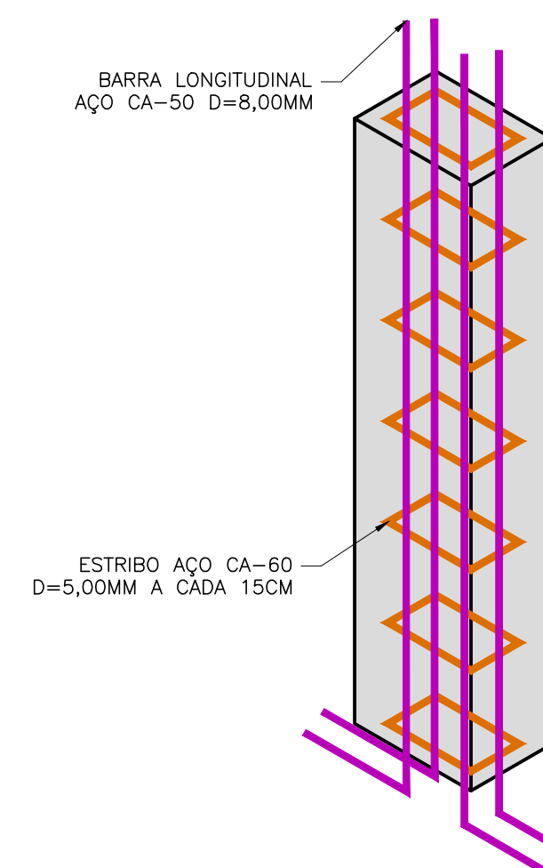
5 DETALHE PILARES 20X14 ESCALA 1:10
