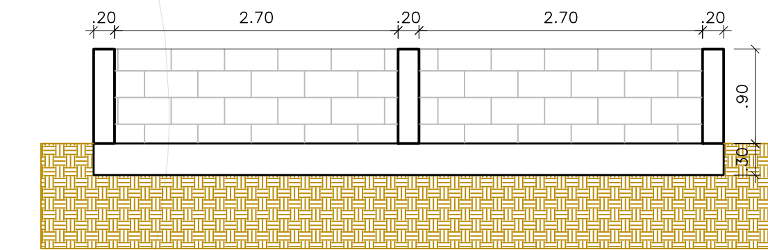
3 DETALHE TIPO MURETA H= 0,9M ESCALA 1:50
