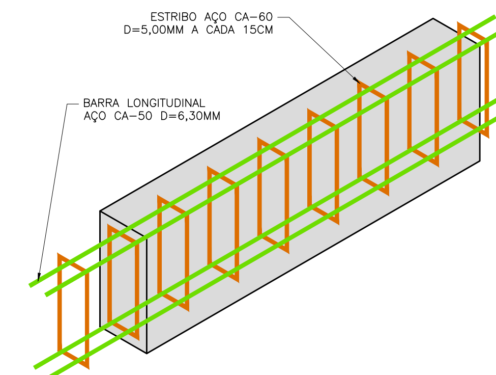
4 DETALHE VIGAS 30X14 ESCALA 1:10
